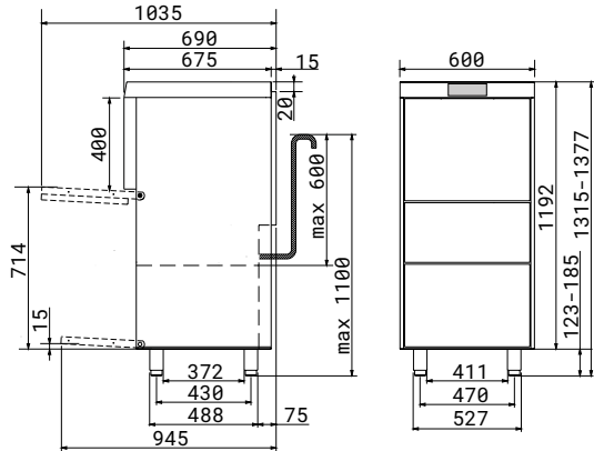
Hood Type 600×500
