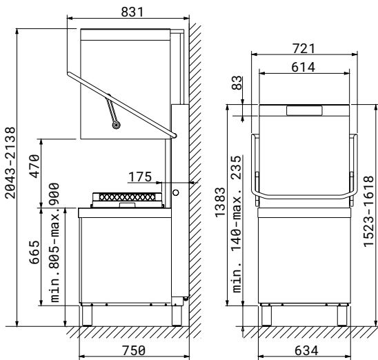
Hood Type 500×500
