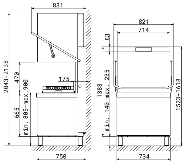
Hood Type 600×500
